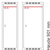
Dybde 400 / 550 mm
