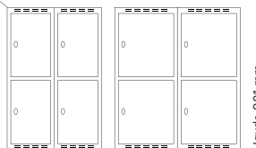
Dybde 400 / 550 mm
