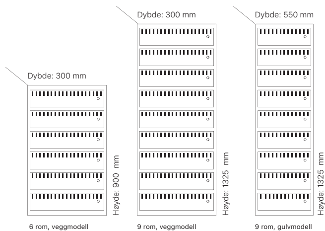
6 rom, veggmodell
