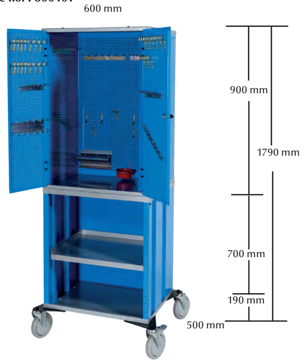
VERKTYGSVAGN, HÅLLARE OCH STICKERS FÖR 105 VERKTYG TOOL TROLLEY, HOLDERS AND STICKERS FOR 105 TOOLS Article no. : 800401
