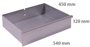
LÅDSATS 1 / DRAWER SET 1 Article no. 800133
