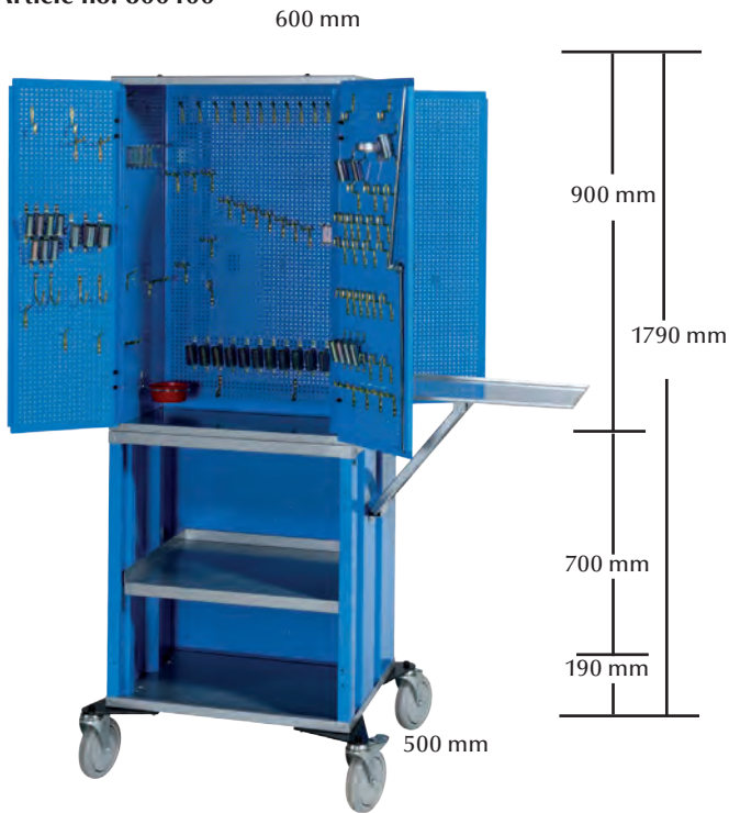
VERKTYGSVAGN, HÅLLARE OCH STICKERS FÖR 154 VERKTYG TOOL TROLLEY, HOLDERS AND STICKERS FOR 154 TOOLS Article no. 800400
